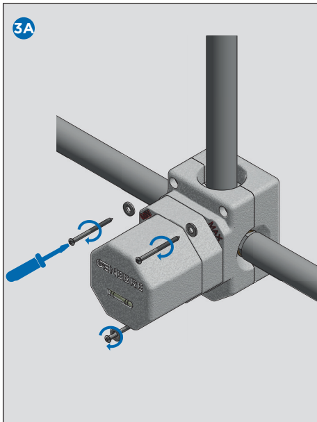
Type 1. Montaje directo Type 1. Direct assembly
