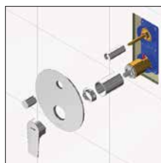
Posteriormente se instala el Kit y la maneta dejando la instalación terminada. The Kit and the handle can be installed, finishing the installation.
