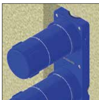
Para indicar la profundidad correcta de montaje dispone de contornos con marcas MAX/MIN. To indicate the correct mounting depth, has contours with MAX/MIN marks.
