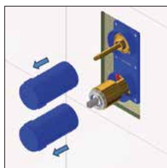
El tapón protector se extrae una vez colocados los azulejos para evitar daños en la grifería. The protective cap is removed once the tiles have been installed to prevent damages to the taps.
